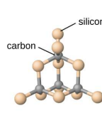
silicon carbide
