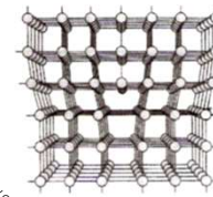
Edge dislocation
